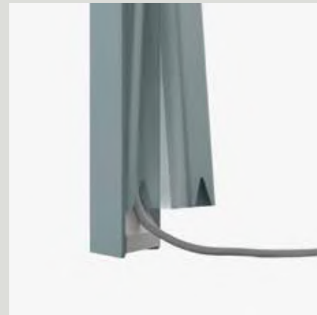
Canale passacavi in lamiera verticale - ispezionabile Vertical sheet metal cable duct - accessible
